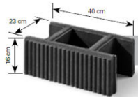
Pustak ryflowany (podmurówkowy) symbol: C2 waga: ok. 15,5 kg
