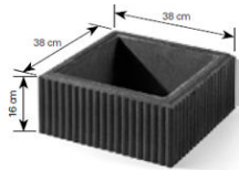
Pustak ryflowany (słupkowy) symbol: C1 waga: ok. 20,5 kg
