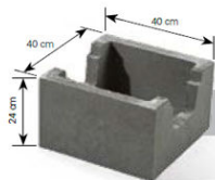
Pustak fundamentowy (z wpustem) symbol: D2 waga: ok. 30 kg
