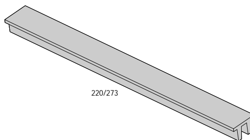
BELKA PODWALINOWA (220 cm) SYMBOL: D3 WAGA: ok. 75 kg
