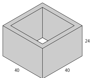
PUSTAK FUNDAMENTOWY SYMBOL: D1 WAGA: ok. 33 kg
