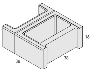
PUSTAK PODMURÓWKOWY SYMBOL: B1 WAGA: ok. 25,5 kg
