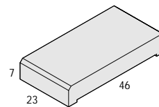
DASZEK PŁASKI SYMBOL: E16 WAGA: ok. 14 kg
