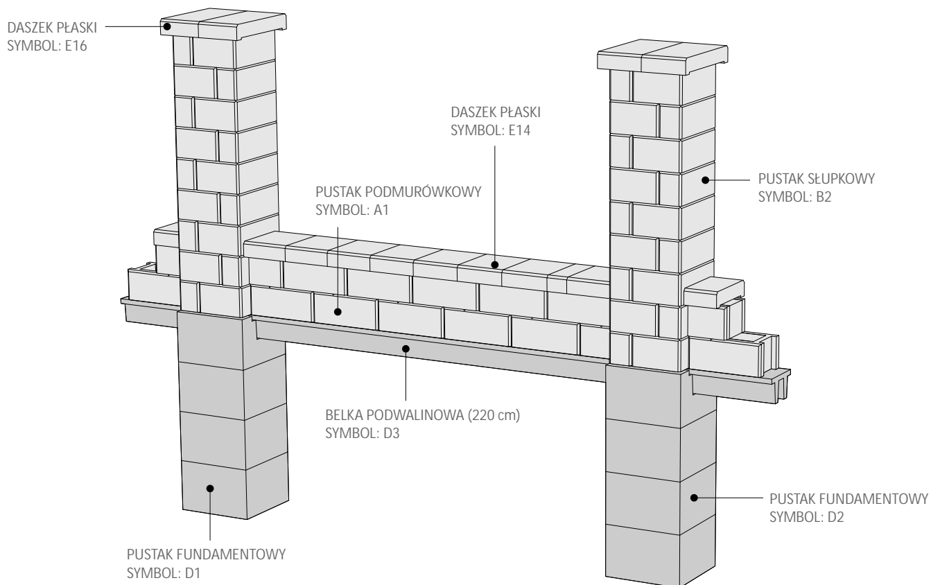
DASZEK PŁASKI SYMBOL: E14 WAGA: ok. 11,5 kg
