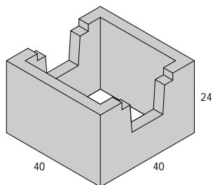
PUSTAK FUNDAMENTOWY SYMBOL: D2 WAGA: ok. 30 kg
