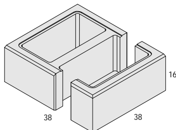
PUSTAK SŁUPKOWY SYMBOL: B2 WAGA: ok. 25,5 kg
